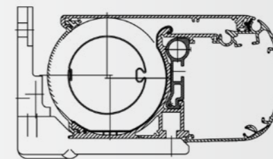
▲ Frontprofil rund
