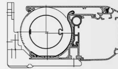
▲ Frontprofil eckig
